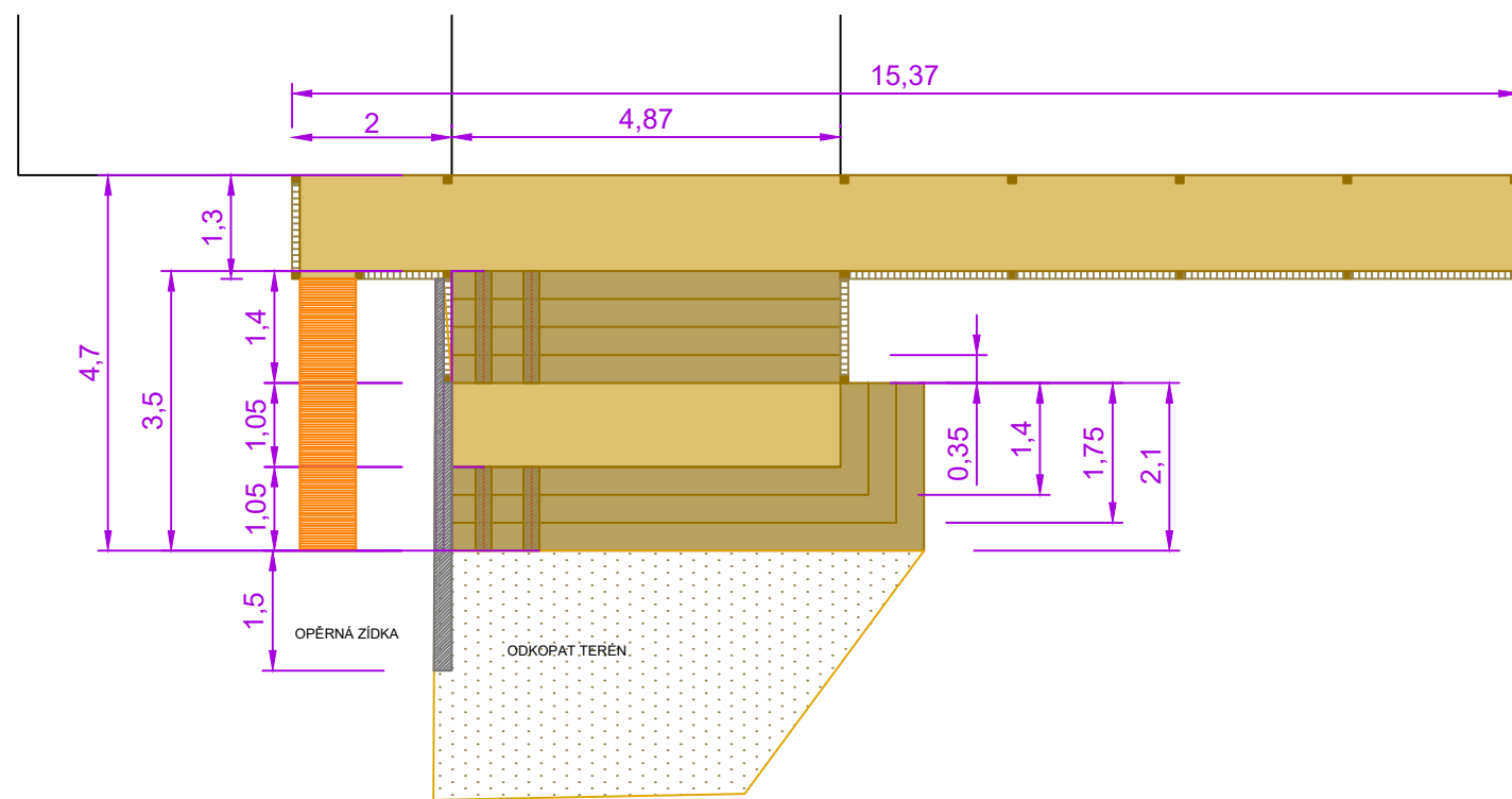
SCHODIŠTĚ NA NÁVES 1 : 100
