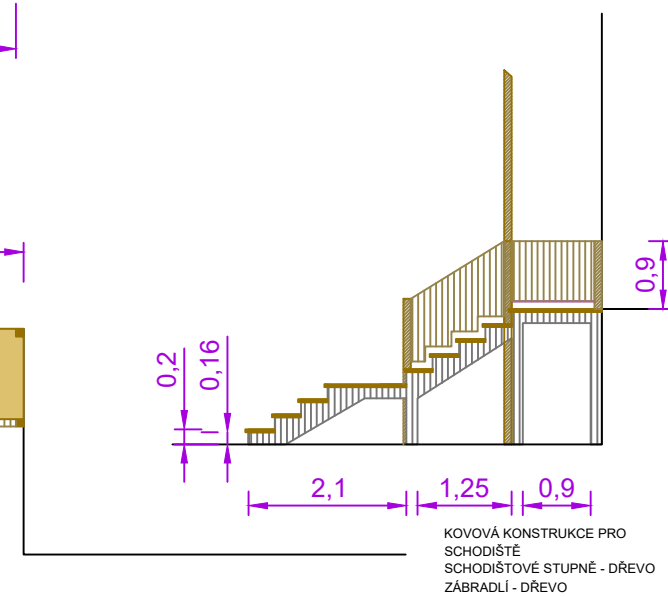
SCHODIŠTĚ NA NÁVES 1 : 100
